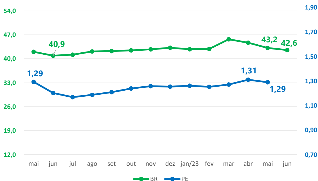
Figura 11 - Consumo de energia elétrica na rede (1 milhão MWh)
